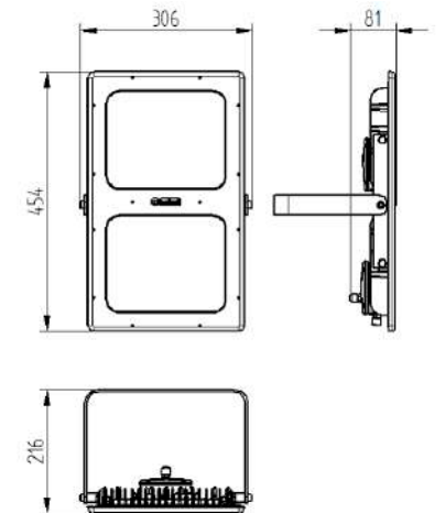
Unidade de medida (mm)
