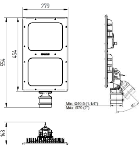
Unidade de medida (mm)
