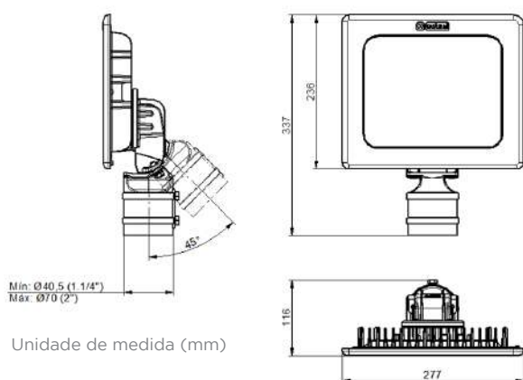
MODELO POSTE ARTICULADO
